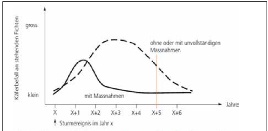
Verlauf einer Borkenkäfer-Massenvermehrung mit und ohne Bekämpfungsmaßnahmen (Sturm- und Käferholzräumung), wie sie nach den Stürmen Vivian (1990) und Lothar (1999) beobachtet werden konnte.
