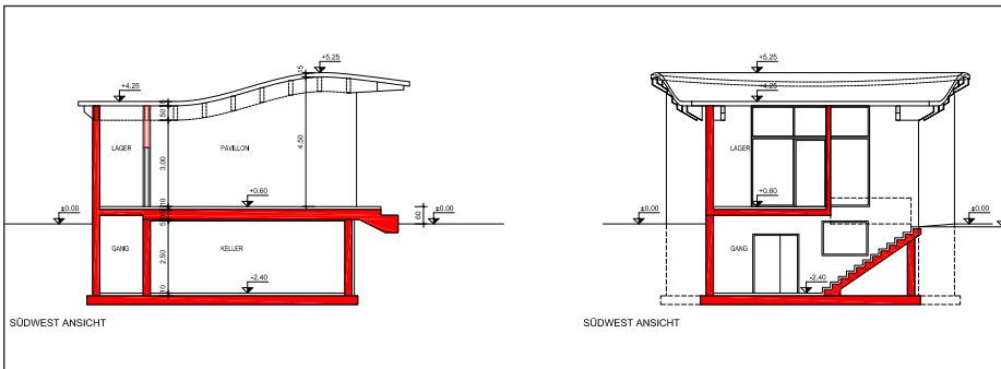
Dorfplatz - Ansichten, Schnitt
