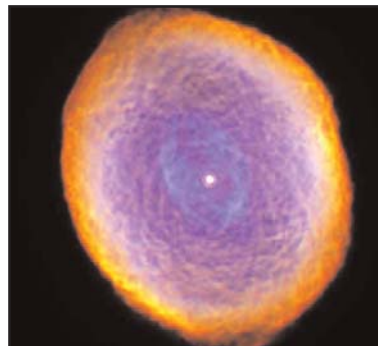
PN 7, ein so genannter Planetarischer Nebel. Diese Gas-Nebel bilden sich um sterbende Sterne. Auch unsere Sonne wird in mehr als 7 Milliarden Jahren einen ähnlichen Nebel abwerfen.
